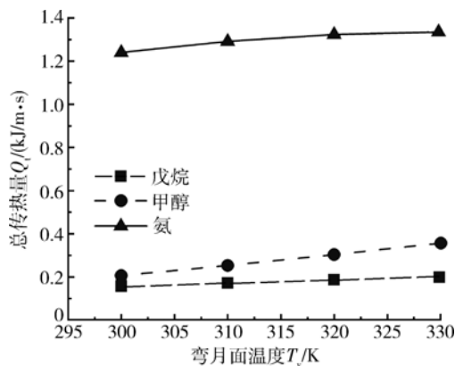
图 7 不同工质总传热量 Q_e 随 T_v 的变化 ( \Delta T=1 K)
