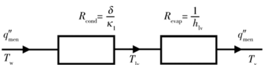
图2 蒸发薄膜热阻关系图
