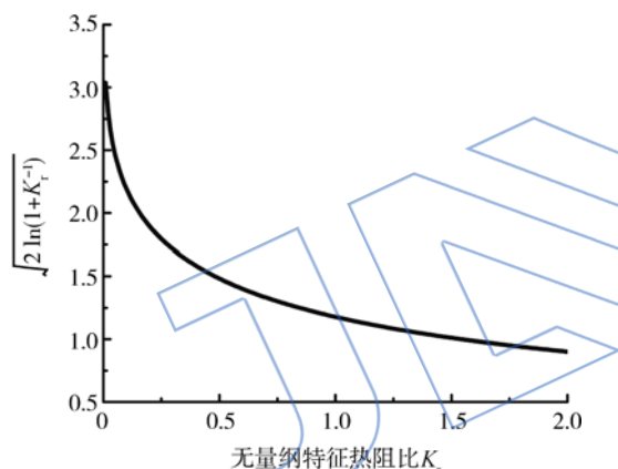
图3 \sqrt{2 \ln(1 + K_r^{-1})} 的值随 K_r 的变化
