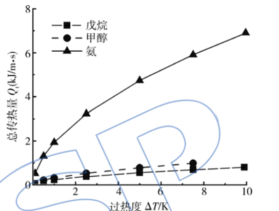
图 8 不同工质总传热量 Q_e 随 \Delta T 的变化 ( T_v=300 K)
