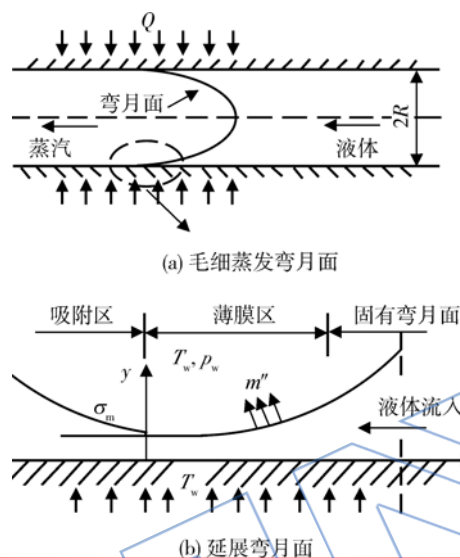
图1 毛细通道内蒸发弯月面分析示意图
